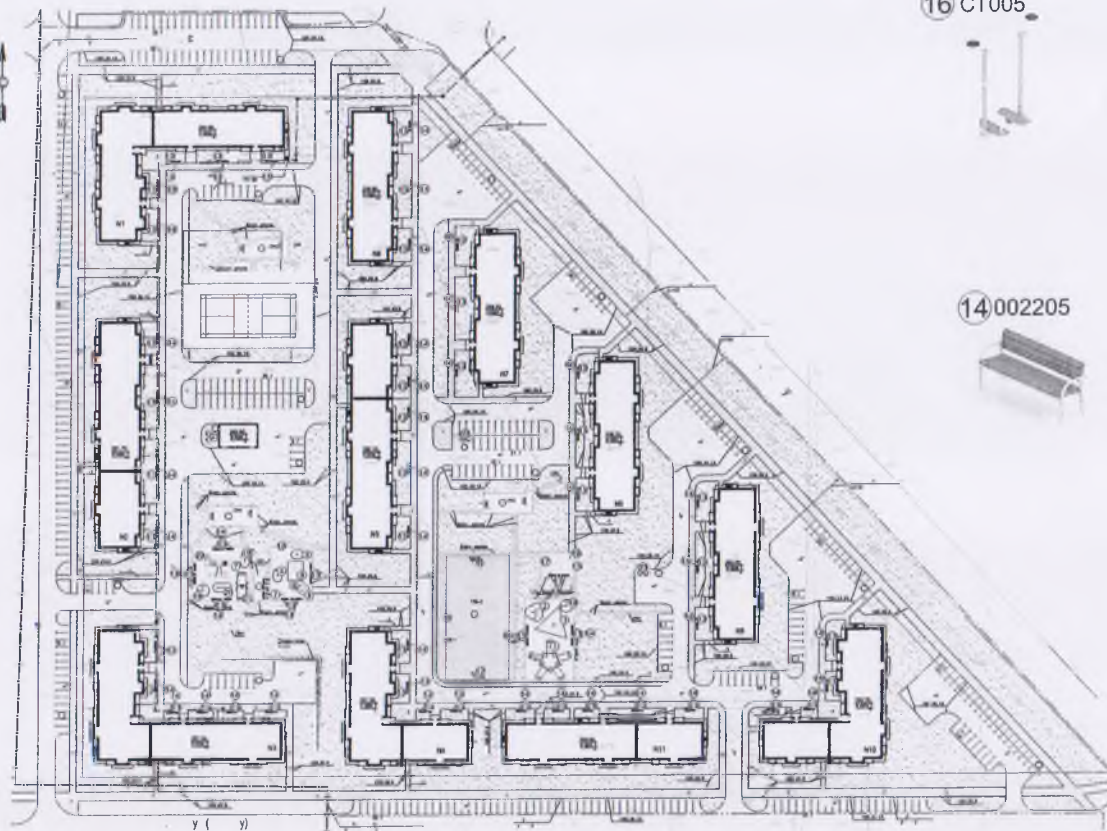
Схема расположения детского игрового и уличного оборудования М 1:500
