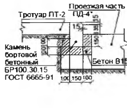
УЗЛЫ ПРИМЫКАНИЯ ПОКРЫТИЙ
